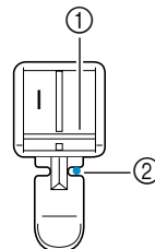
① Стержень на правой стороне лапки ② Точка опускания иглы
