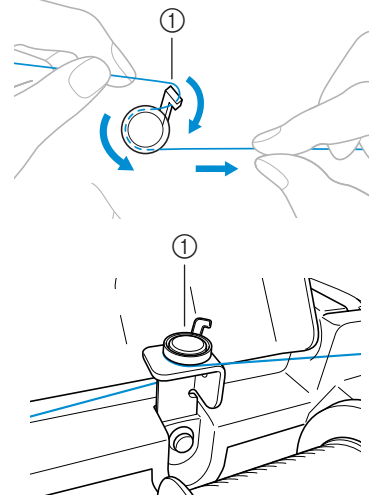
① Направляющая нити для намотки шпульки
