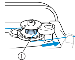
① Прорез в седле устройства намотки шпульки
