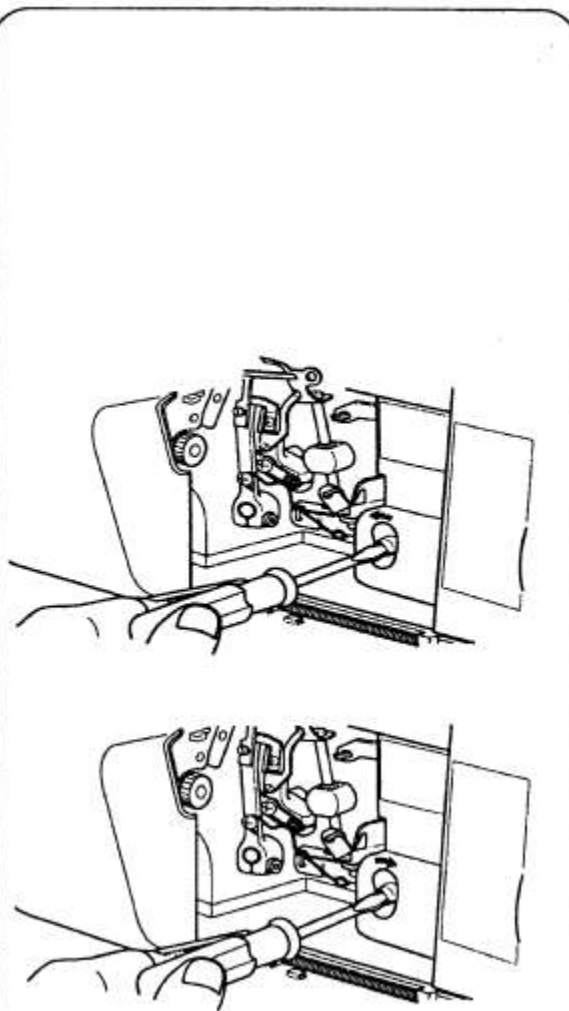
Крышка ножа
