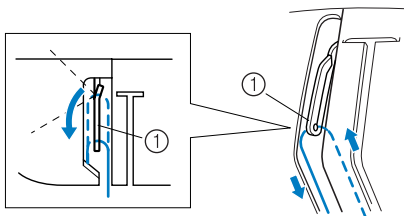
① Рычаг нитепритягивателя
